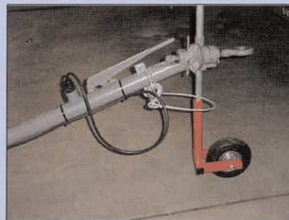
Dès que le dispositif est en place, une personne peut facilement déplacer la remorque ou la moto-pompe
