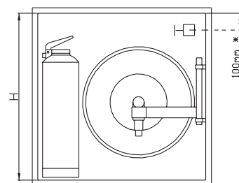
Ausführung UP Art. Nr. 10.20454UP40
