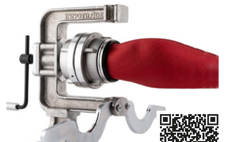
INNOTRADE-Montagegerät.
